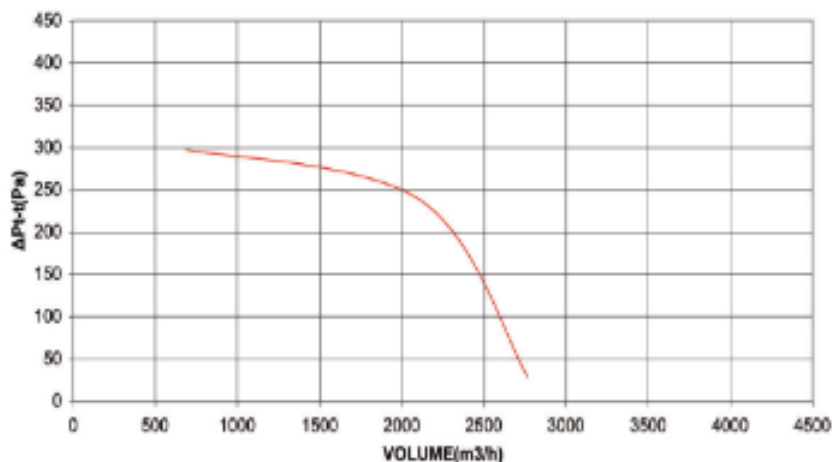
Φ200-0.5HP-1450RPM
