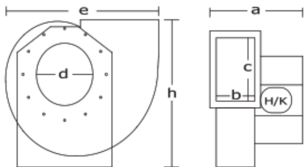
Φ200-0.5HP-1450RPM
